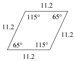
rhombus
