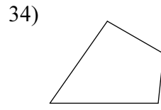
quadrilateral
