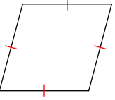
rhombus
