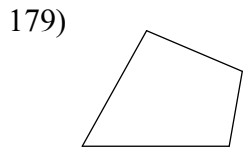
quadrilateral
