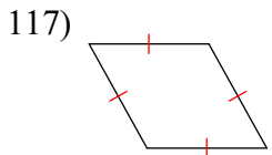
rhombus
