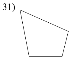
quadrilateral
