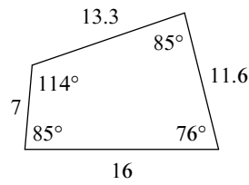
quadrilateral
