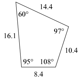
quadrilateral
