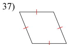
rhombus
