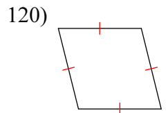
rhombus
