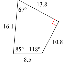
quadrilateral
