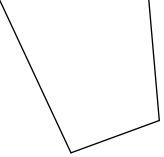
quadrilateral
