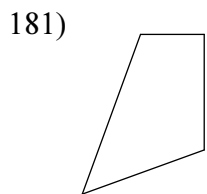
quadrilateral
