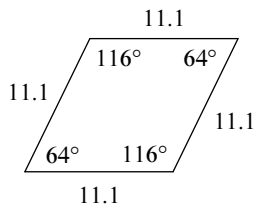
rhombus
