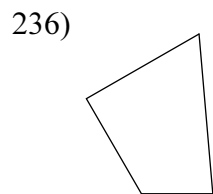
quadrilateral
