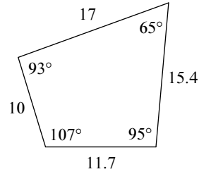
quadrilateral
