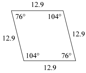
rhombus
