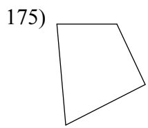
quadrilateral
