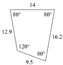
quadrilateral
