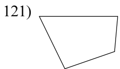
quadrilateral
