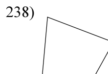
quadrilateral
