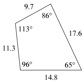
quadrilateral
