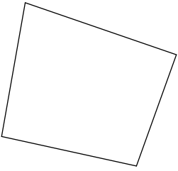
quadrilateral
