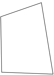
quadrilateral
