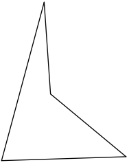
quadrilateral
