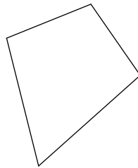
quadrilateral
